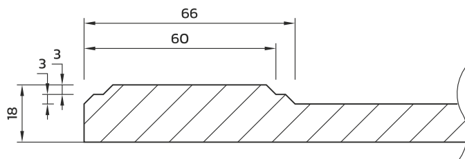
PRZEKRÓJ
