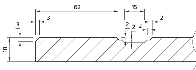
PRZEKRÓJ
