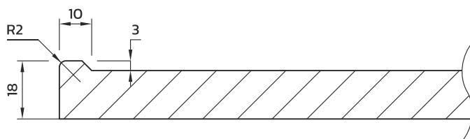
PRZEKRÓJ
