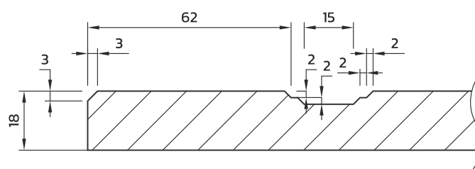
PRZEKRÓJ
