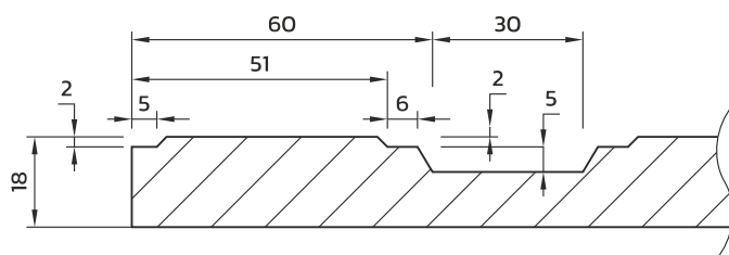
PRZEKRÓJ
