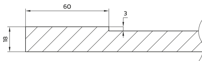
PRZEKRÓJ
